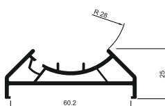
Профиль адаптера к трубе Арт. 6013
