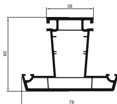
Профиль импоста Арт. 6003
